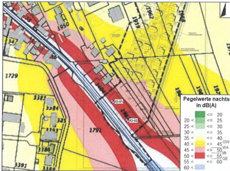
Abbildung 3 - Pegelverteilung nachts, Rechenhöhe 8 m über Gelände
