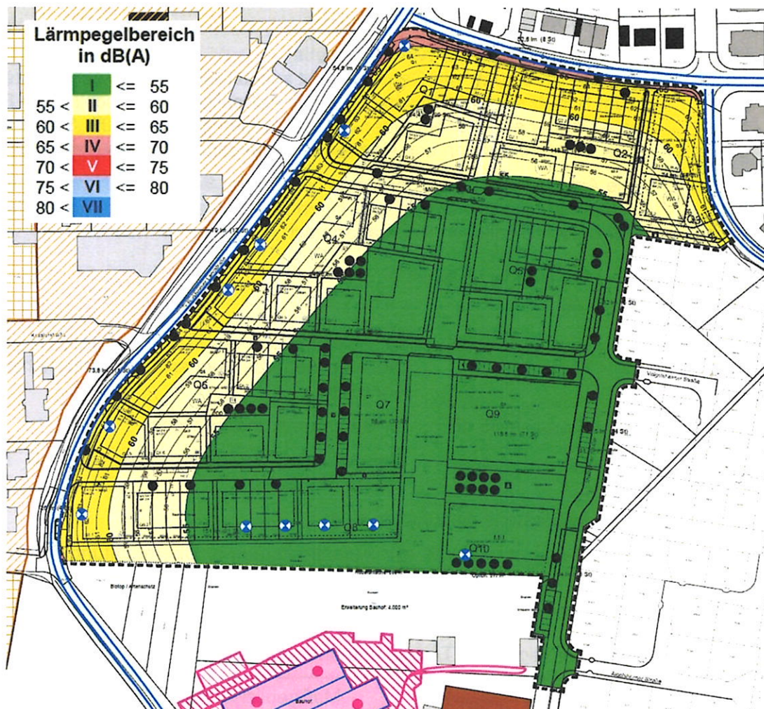
Lärmpegelbereiche gemäß DIN 4109-1 (2018) (Quelle: Büro Heine + Jud, Stand: 12.12.2023)
